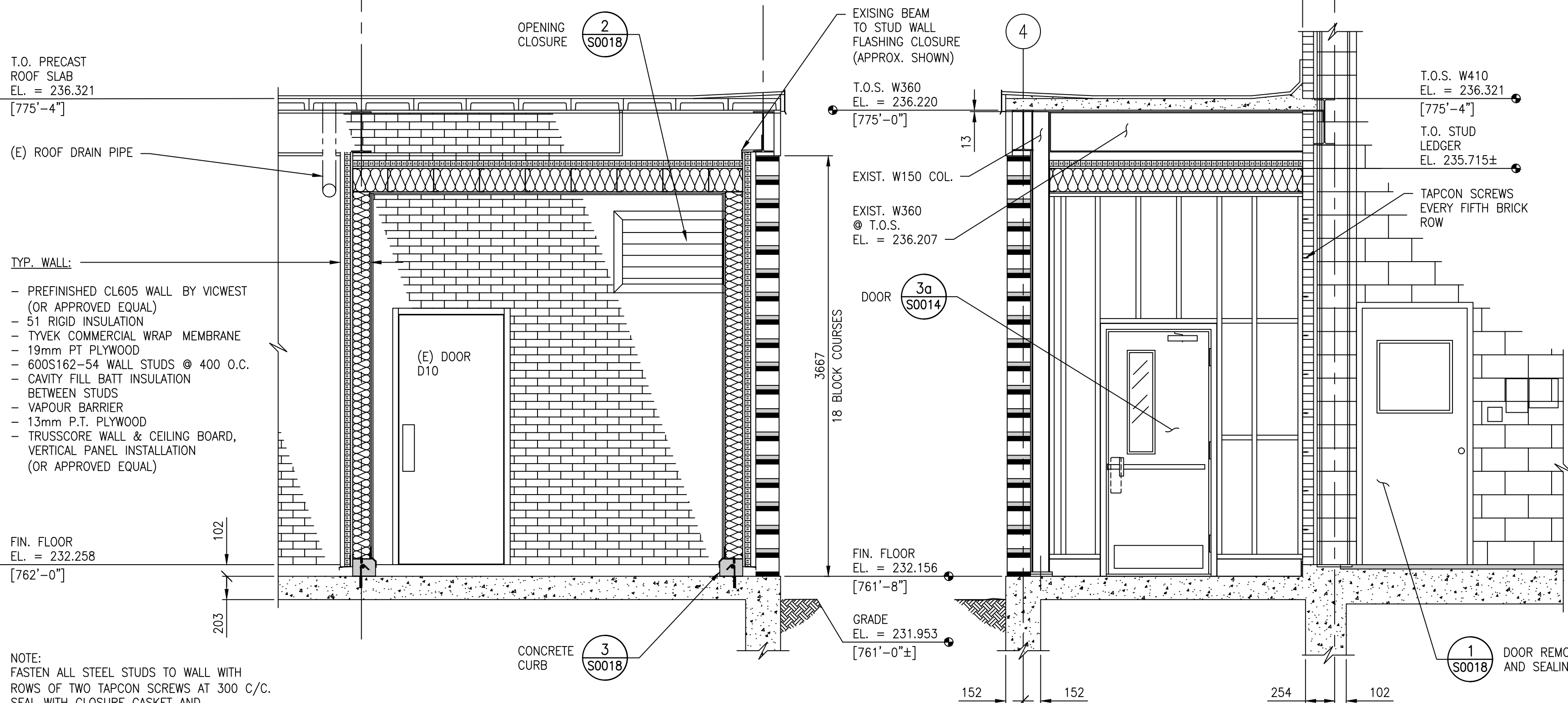
SECTION A SCALE: 1 : 30
